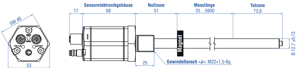
Abb. 2: Temposonics® RH5 mit Ringmagnet
